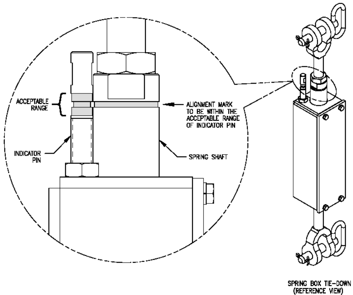
Figure 4.3.1-2 – TRUPACT-III Tiedown
